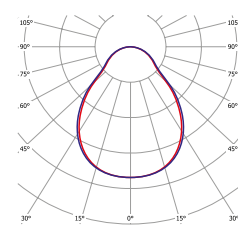
— C0 - C180 — C90 - C270 P2
