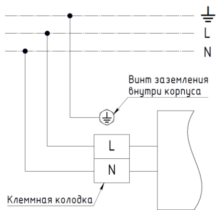
Схема подключения.
