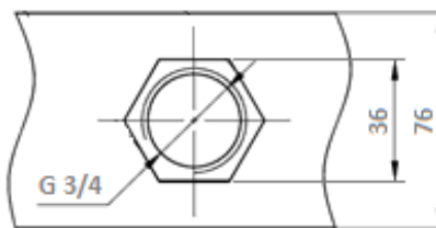
СКОБА С МУФТОЙ ДЛЯ УСТАНОВКИ НА ТРУБУ ВАРИАНТ 2
