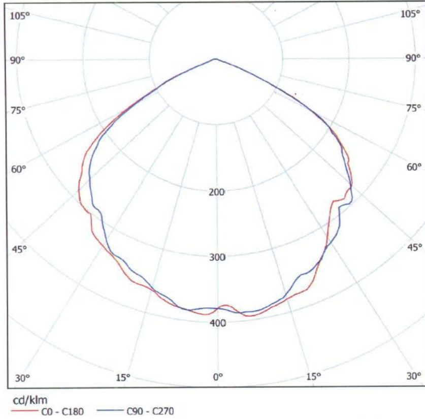
Кривые распределения силы света в 2 плоскостях светильника светодиодного взрывозащищённого ДСП 48-80-БЗ-СП-01, УХЛ1, IP65
