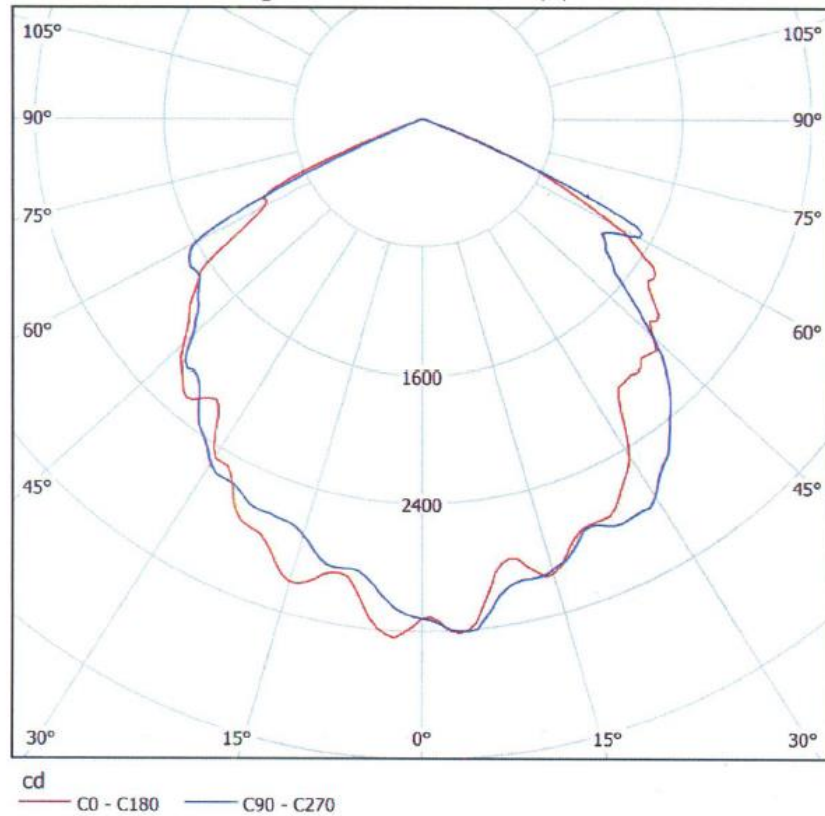
Кривые распределения силы света в 2 плоскостях светильника светодиодного взрывозащищённого ДСП 48-60-БЗ-СП-01, УХЛ1, IP65
