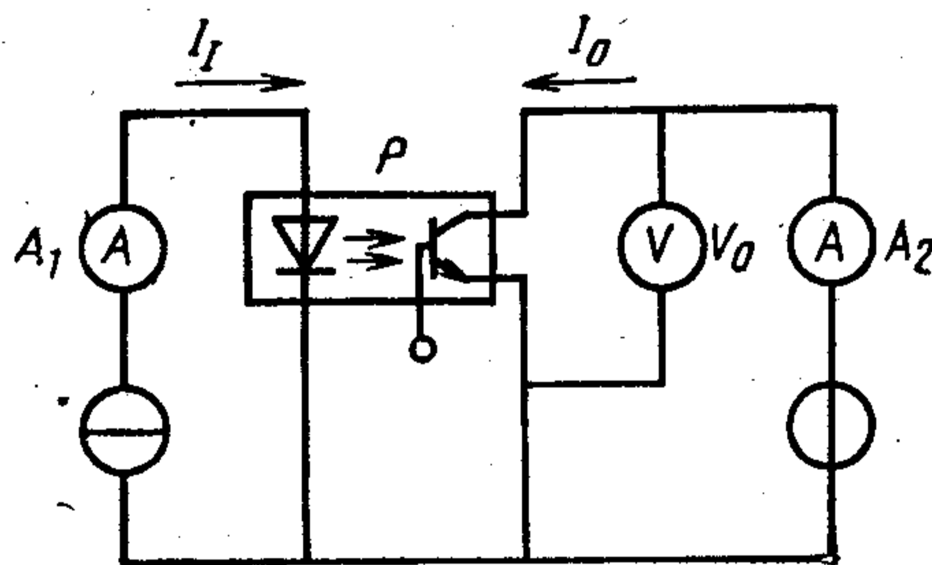
Принципиальная схема
